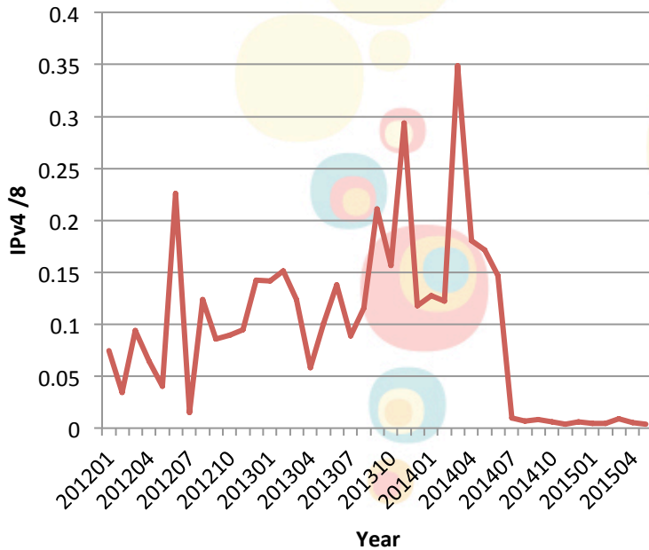
IPv4 /8 per Year
